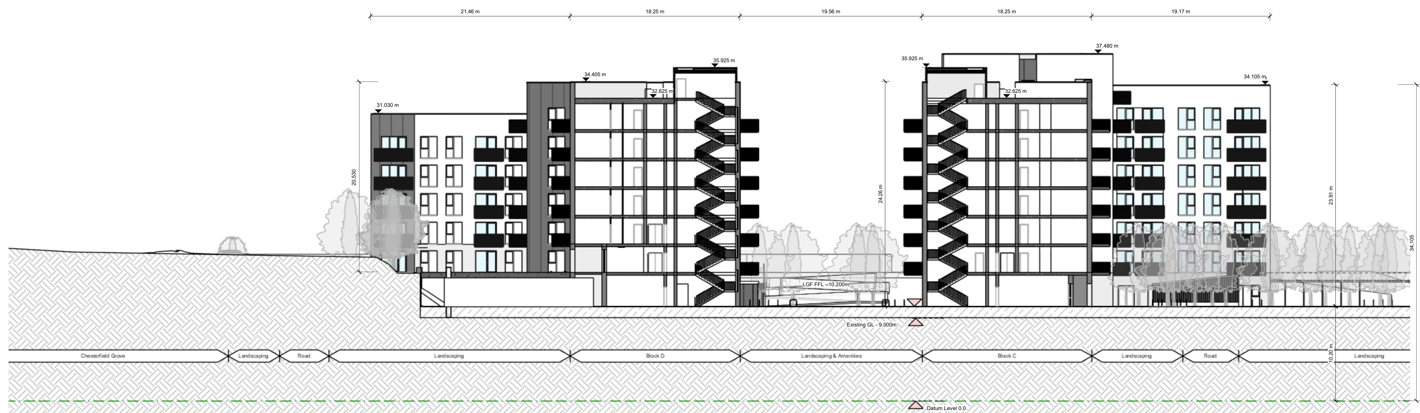
Site Section B-B 1:200
