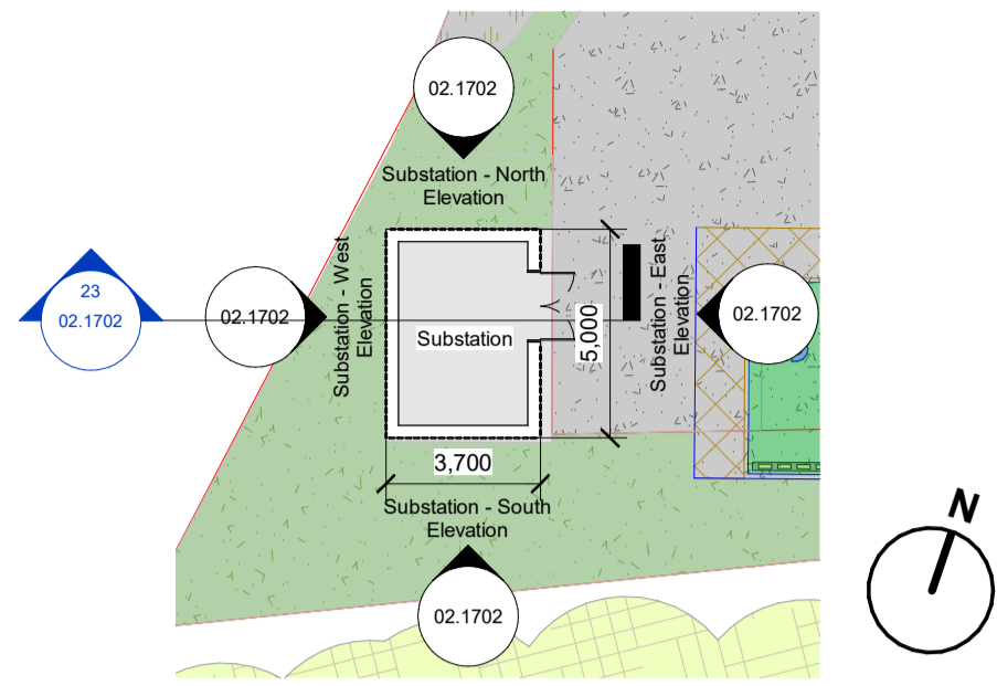
L00 - Site Plan - Substation 1 : 200
